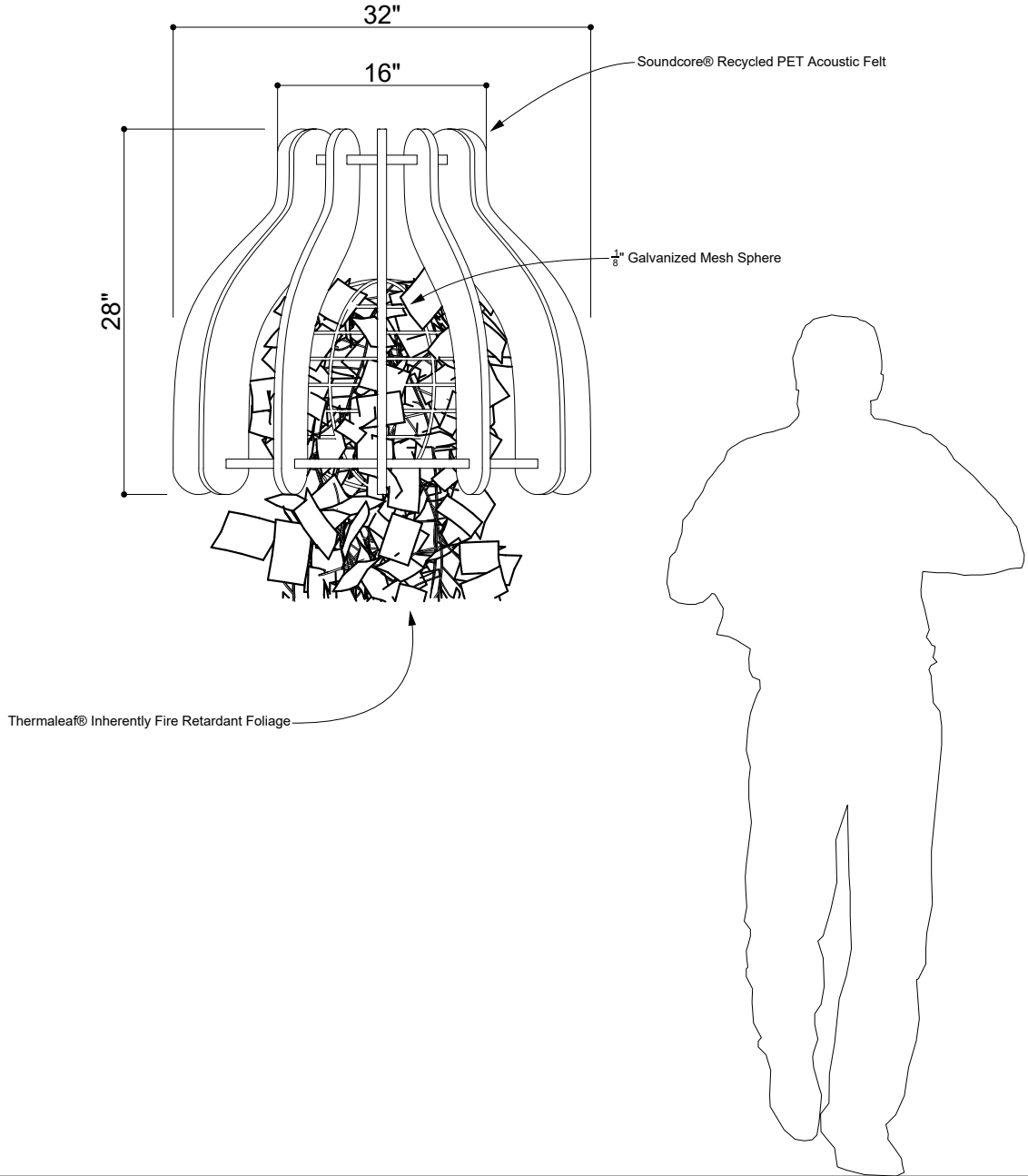
① ELEVATION 1
